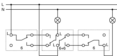
Comutator cap scară cu comutator dublu
