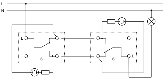
Comutator cap scară
