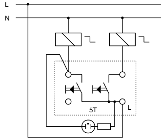
Buton dublu (cu 2 contacte ND)
