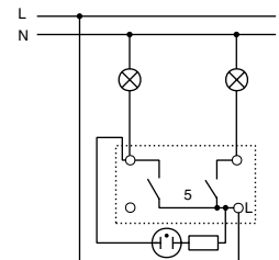
Înterupător dublu / semnalizat cu LED
