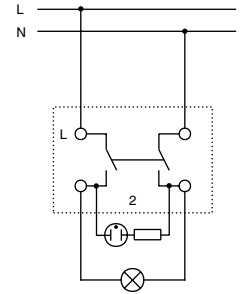
Înterupător cu semnalizare de control, 2-poli
