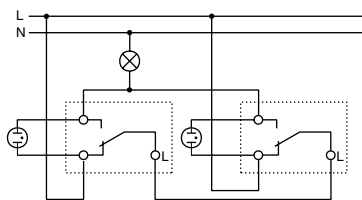
Comutator cap scară luminos, schemă economică
