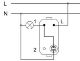
Înterupător cu semnalizare de control, 1-pol
